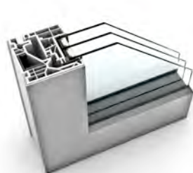
KF 520 PROZOR PVC/ALUMINIJ
