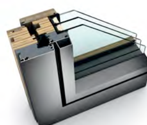
HF 410 PROZOR DRVO/ALUMINIJ
